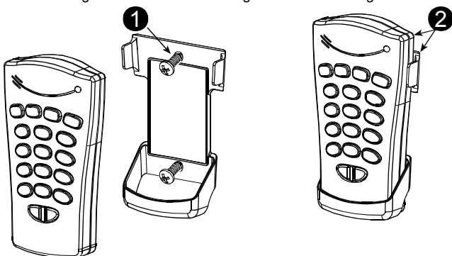
Abb. 2 - Montage
